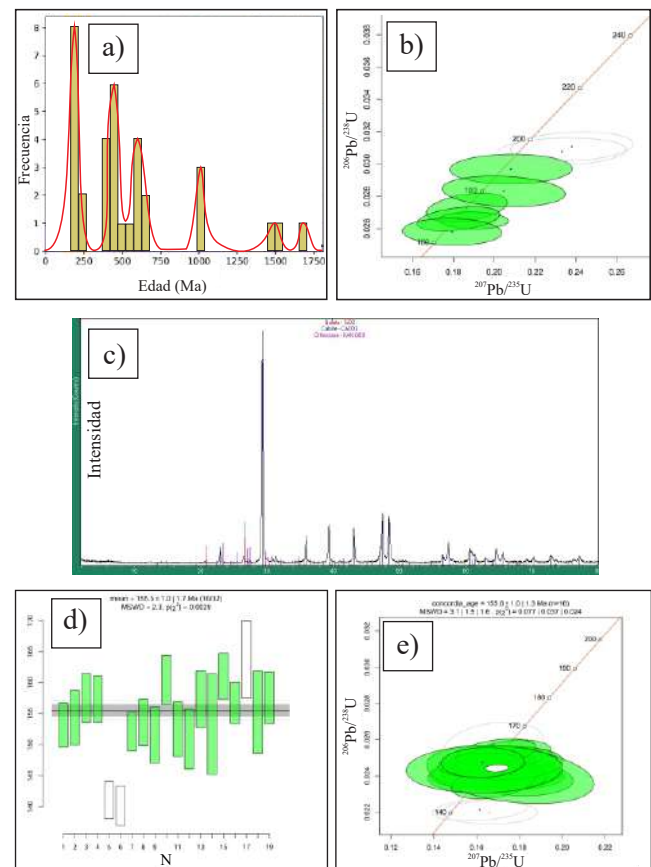
Figura 8. Geocronología U-Pb en circones de la base de la Formación Olvido (a, muestra JP 125-02) y miembro medio (d, muestra JP 125-03). Diagramas de concordia respectivos (b y e). Difractograma de rayos X (c, muestra JP 125-03). Descripción en el texto.
