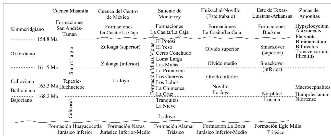
Figura 11. Correlación estratigráfica regional de las formaciones del Jurásico Medio–Jurásico Superior. Líneas onduladas representan discordancias.
