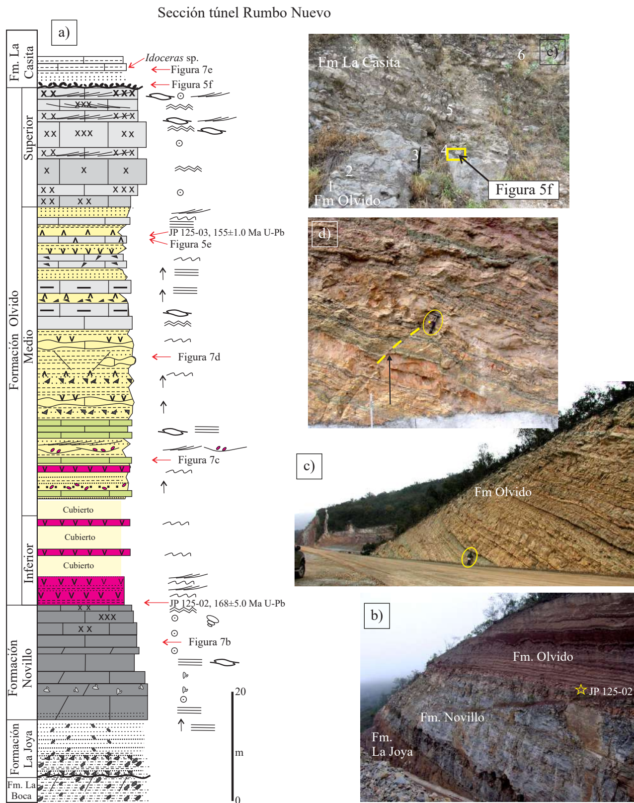
Figura 7. Sección estratigráfica túnel Rumbo Nuevo, kilómetros 25.5 y 27.980 de la carretera del mismo nombre. Ver leyenda en la Figura 3. Descripción en el texto.
