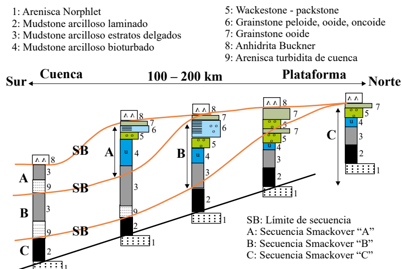
Figura 12. Modelo estratigráfico de secuencias genéticas de la Formación Smackover (tomado de Heydari y Baria, 2006, modificado en este trabajo).
