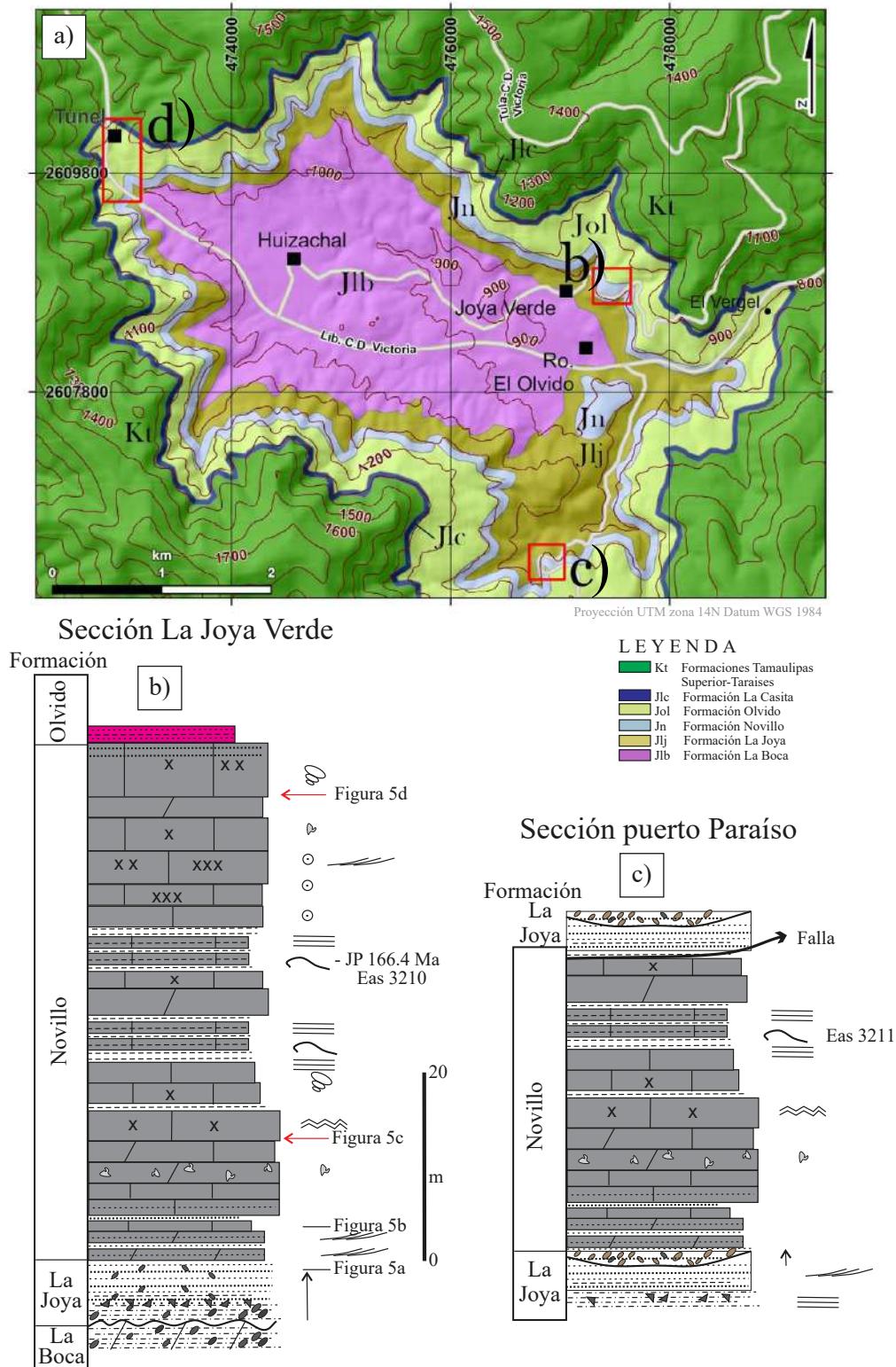
Figura 4. Mapa geológico del valle del Huizachal (a). Los recuadros rojos indican la ubicación de las secciones estratigráficas La Joya Verde (b), puerto Paraíso (c), y túnel Rumbo Nuevo (d). Base topográfica de INEGI F14A29, escala 1:50000. Sección estratigráfica medida en la localidad La Joya Verde (b) y puerto Paraíso (c). Ver leyenda en la Figura 3. Descripción en el texto.
