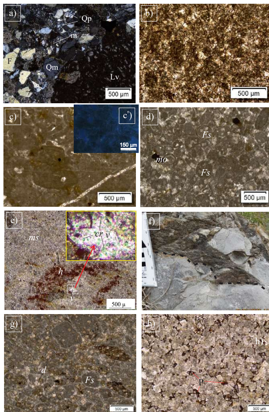
Figura 5. Petrografía de muestras en las formaciones Novillo y Olvido. a) Litarenita con granos de cuarzo monocrystalino (Qm), líticos volcánicos (Lv), cuarzo policristalino (Qp), feldespato (F), en matriz arcillosa (m), cemento calcáreo y minerales opacos, en el contacto transicional entre la Formación La Joya y la Formación Novillo (nicols cruzados); b) wackestone de peloides, arcilloso y dolomitizado; c) grainstone oncolítico, con epifluorescencia (c') hay contenido pobre de querógeno; d) caliza grainstone de ooides (cf. Favreina salivensis Fv) y minerales opacos (mo), cerca del contacto con la Formación Olvido; e) caliza mudstone (ms) con cristales de circón (cr) incluidos en vidrio (v) amorfo (en recuadro superior derecho) y hematita (h) luz natural, en el miembro medio de la Formación Olvido (muestra JP 125-03); f) Detalle de la superficie de erosión rellena por brecha en el contacto de las formaciones Olvido y La Casita; g) caliza grainstone de ooides (cf. Favreina salivensis Fs), parcialmente dolomitizada (d), con minerales opacos; h) macrolitolomía con porosidad intercrystalina (P).
