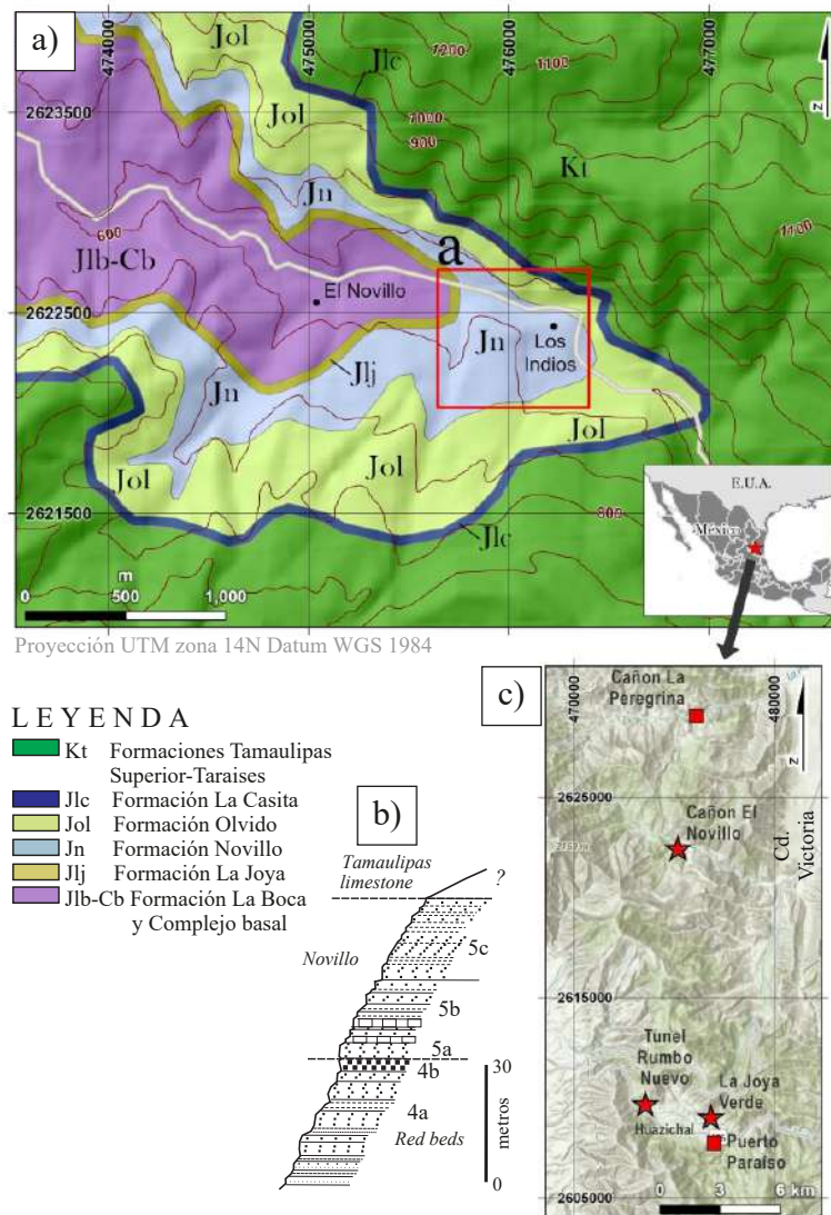
Figura 1. Mapa geológico del cañón del Novillo (a). El recuadro rojo indica la ubicación de la sección estratigráfica El Novillo. b) Sección estratigráfica publicada por Heim (1940), con las litologías 4a – 5c que reconoció, redibujada en este trabajo. c) Mapa con la ubicación regional de las secciones descritas en este trabajo, las estrellas son localidades tipo y los cuadros son localidades adicionales.
