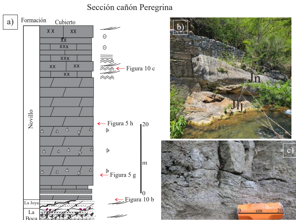
Figura 10. Sección estratigráfica en el cañón Peregrina (a). Contacto estratigráfico (b) entre las formaciones La Joya (Jl) y Novillo (Jn). Carpetas microbianas (c). Ver leyenda en la Figura 3. Explicación en el texto.
