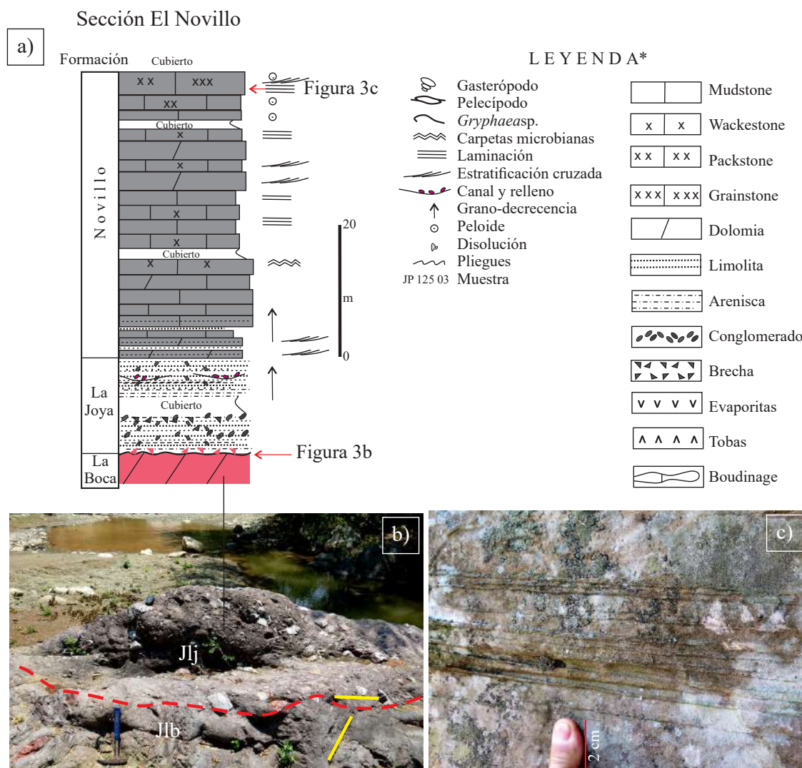
Figura 3. a) Sección estratigráfica en el cañón del Novillo. b) Contacto en discordancia erosiva (línea de color rojo) y angular (líneas de color amarillo) entre las formaciones La Boca (Jlb) y La Joya (Jlj). c) Laminación paralela en la cima de la Formación Novillo (c). *Leyenda para todas las secciones estratigráficas. Descripción en el texto.
