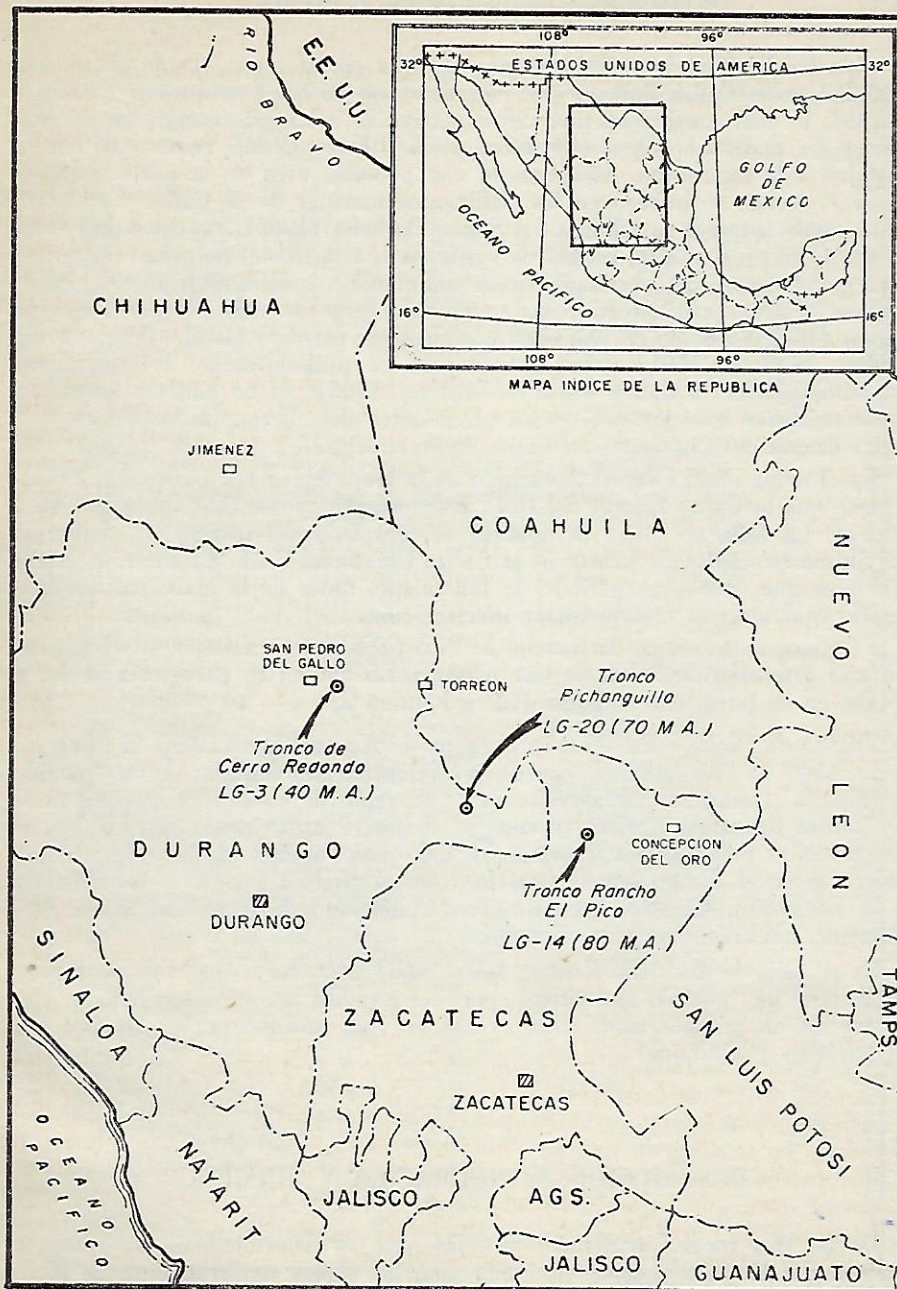
Fig. 1. Mapa índice de la parte centro-septentrional de México que muestra la procedencia y edad, en millones de años de las tres muestras analizadas.
